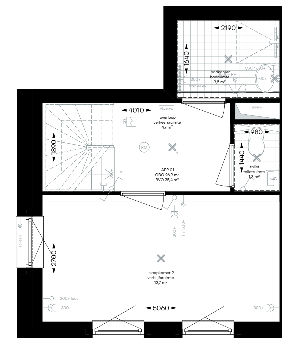
1:50 1e verdieping
