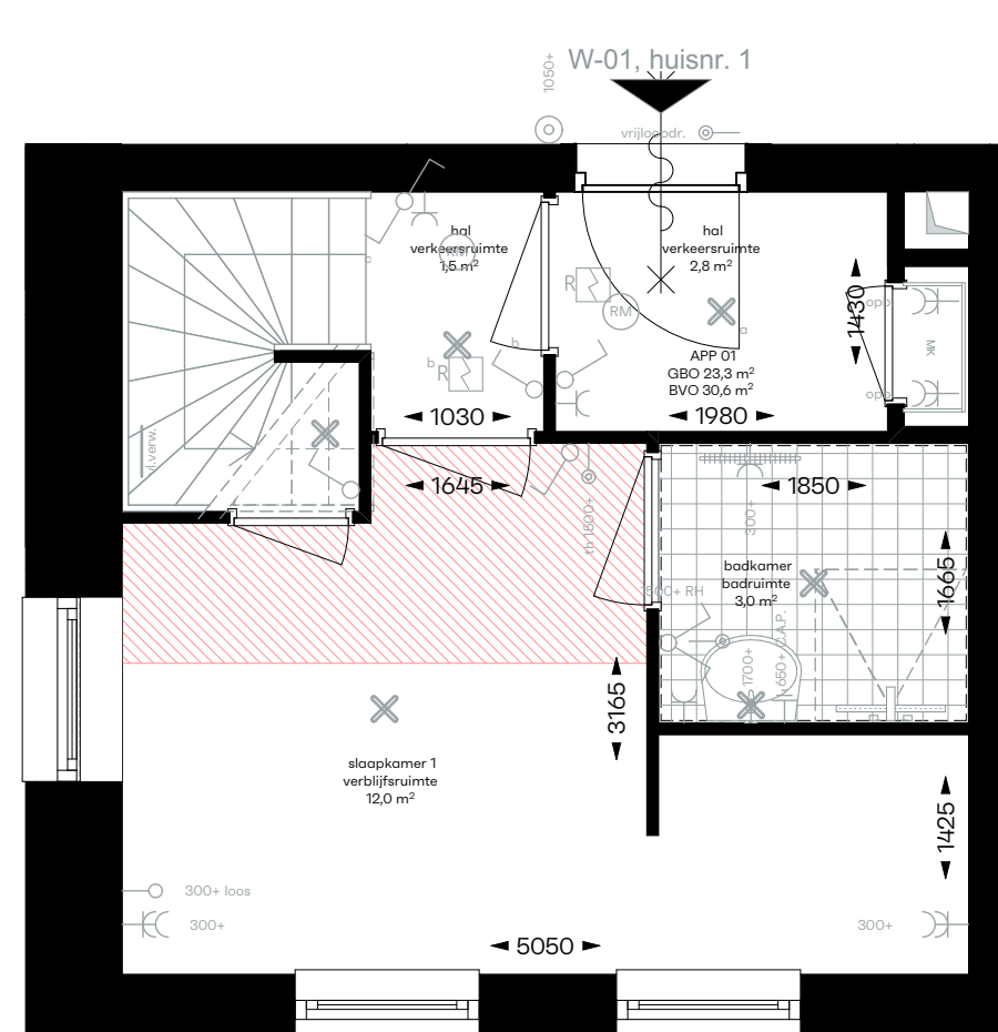
1:50 Souterrain
